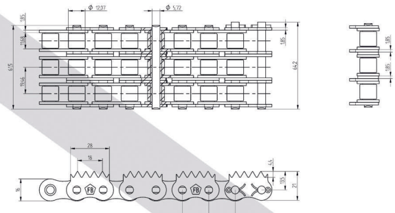
12B-3FBVERZAHNTS6/SO
