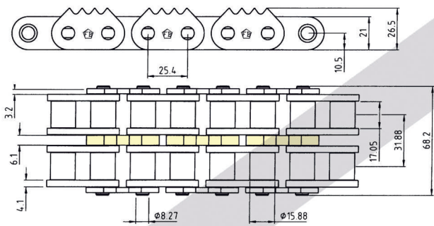
5218.000.18FB / ISO 16B-2 Triplex 5318.000.06 / ISO 16B-3
