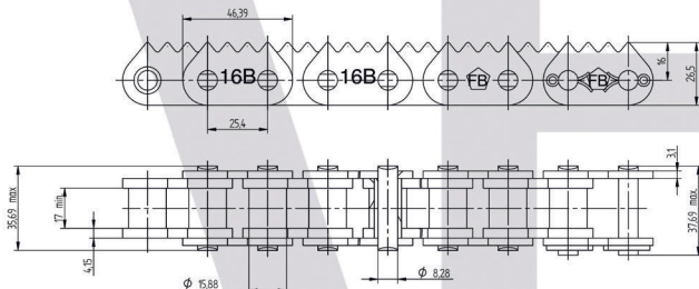
16B-1FBVERZAHNT
