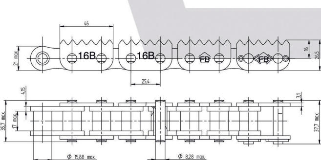
16B-1FBVERZAHNT6x50,8
