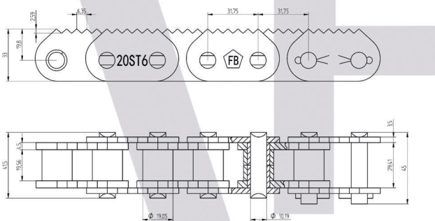
5130.000.22FB
