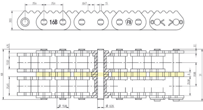
5218.000.19FB / ISO 16B-2 Simplex 5118.000.35 / ISO 16B-1 Triplex 5318.000.07 / ISO 16B-3
