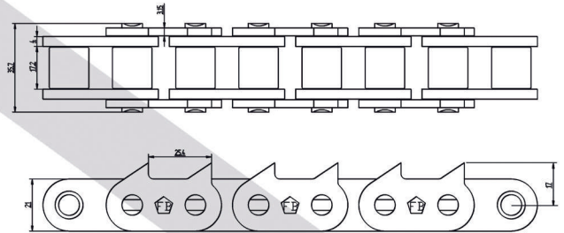
16B-1FBSÄGEVERZ2X50
