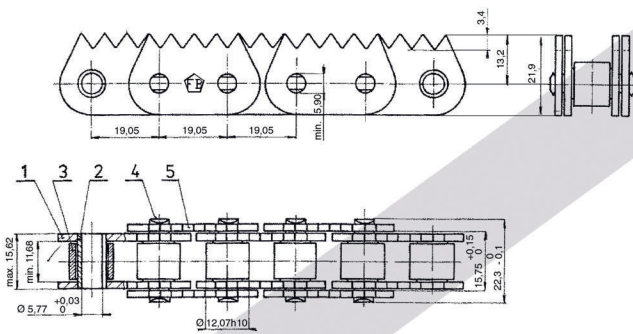
12B-1FBVERZAHNTS5 Duplex 12B-2FBVERZAHNTS5
