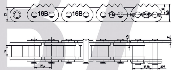
16B-1FBVERZAHNTx50,8 / 5118.000.34
